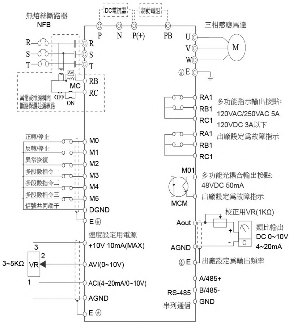
220V 15HP-25HP/440V 20HP-40HP 接線圖
